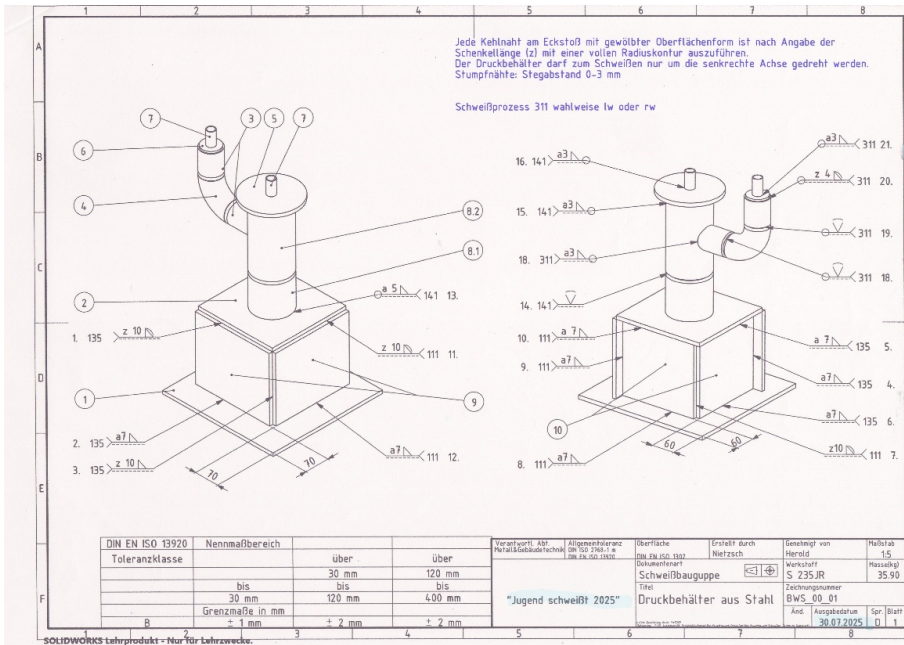
Bild 2: Gruppenaufgabe Druckbehälter
